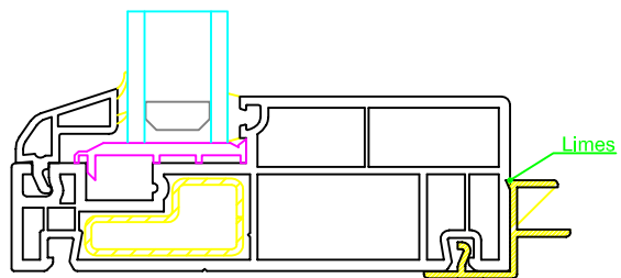
Clipsbar U-Liste - forsat ind, for 10mm plade Notprofil 4
