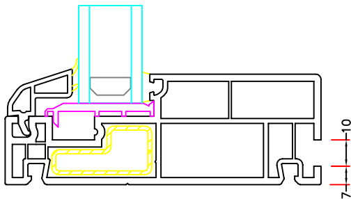
Fræset not i karm
