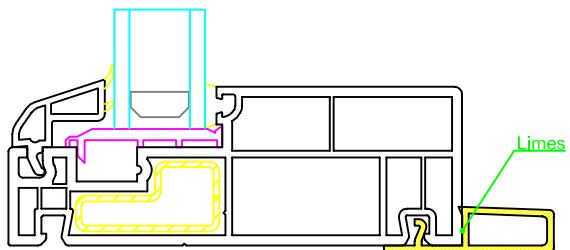
Clipsbar 25mm Karpåforingsliste, for 10mm plade Profil 5
